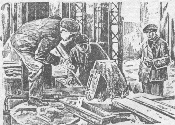
На снимке: первая ванна, из которой получена первая партия советского магния
