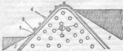
1—Теплоизоляция; 2—оболочка ее; 3—каналы для охлаждения; 4—трубы для дождевания; 5—песок, ил, глина и т. п. материалы
