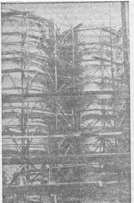
Невхимкомбинат. Монтаж башен
