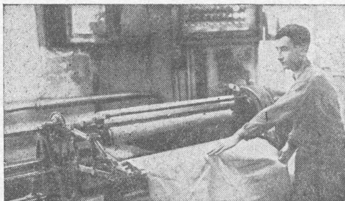
Намотка в рулоны подкладочного материала. Резка матери- рии на любую ширину производится в несколько минут
