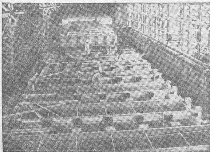
Невхимкомбинат. Насосное отделение. Холодильники
